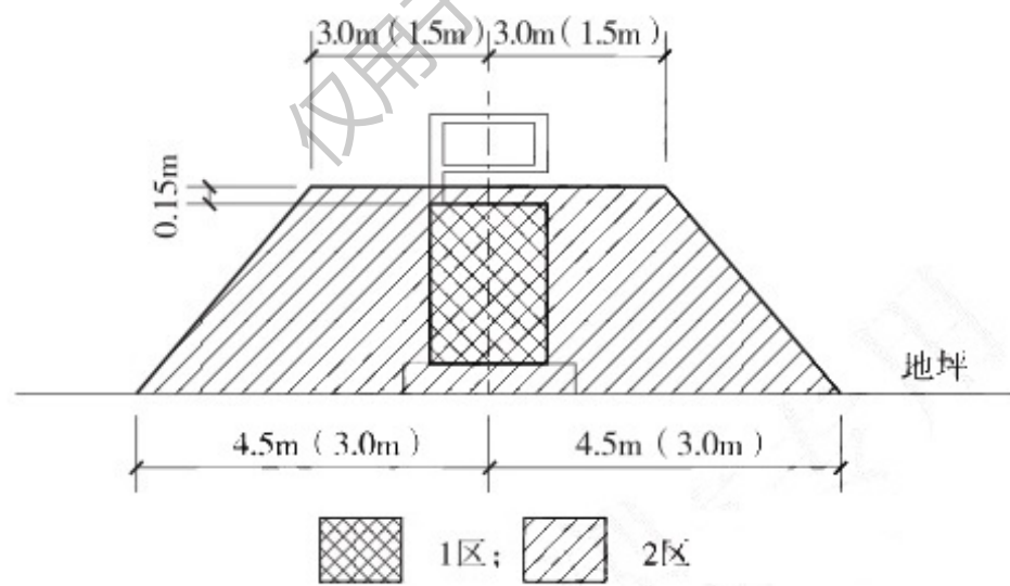
图 3.4-3 汽油加油机爆炸危险区域划分
