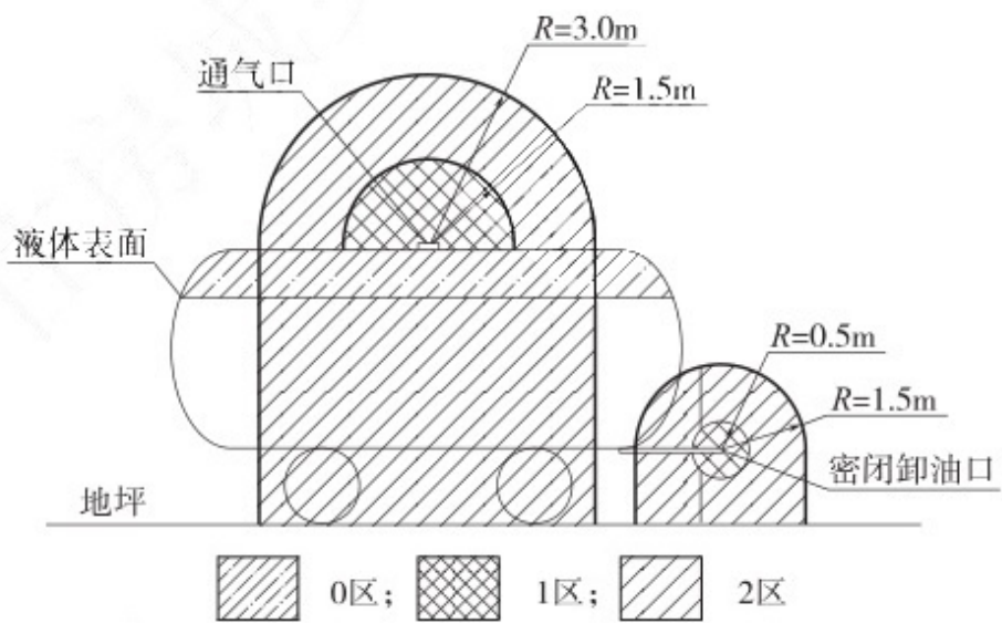
图 3.4-2 汽油油罐车爆炸危险区域划分
