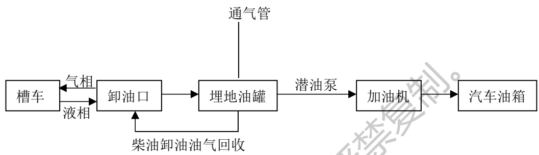
图 2.2-2 柴油工艺流程简图
