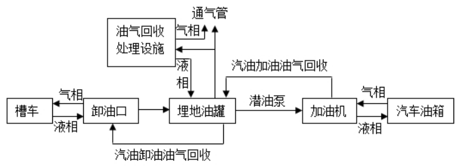
图 2.2-1 汽油工艺流程简图
