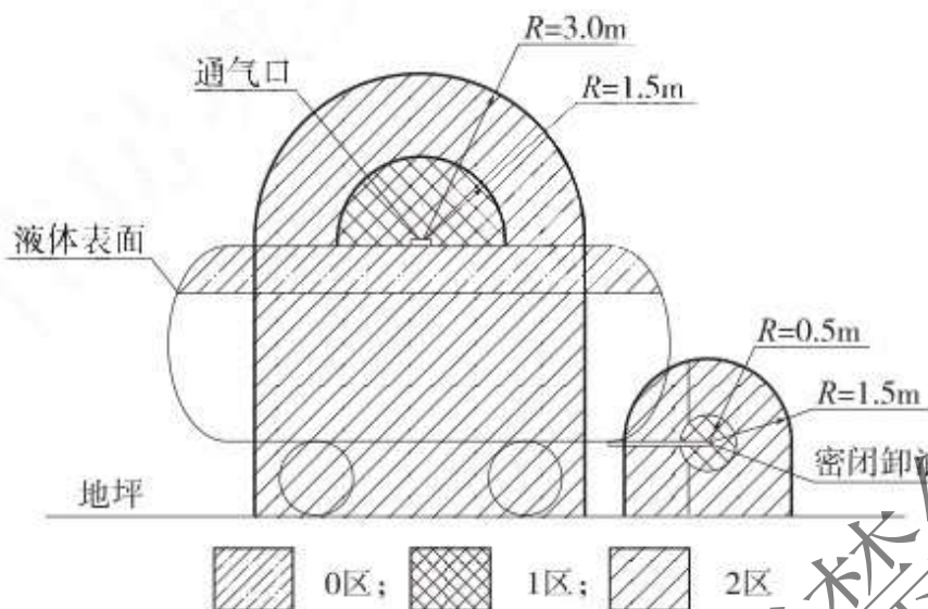
图 3.4-2 汽油油罐车爆炸危险区域划分
