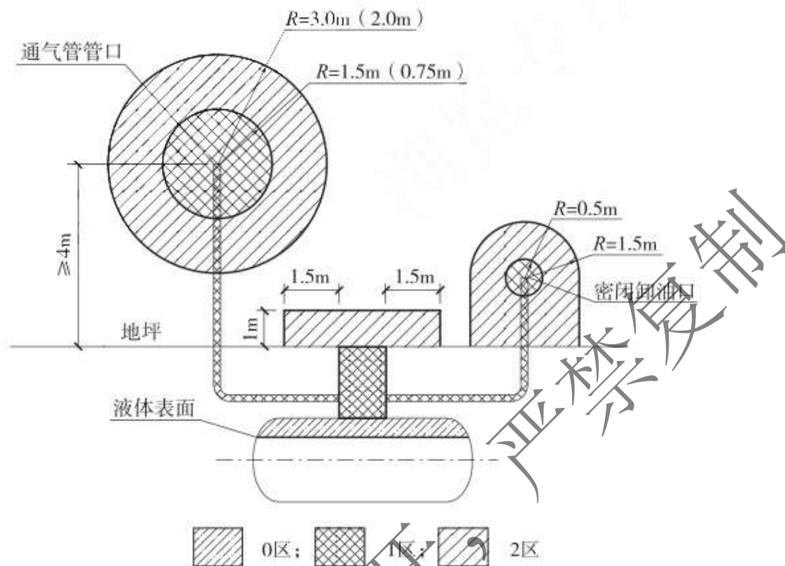
图 3.4-1 汽油埋地卧式油罐爆炸危险区域划分
