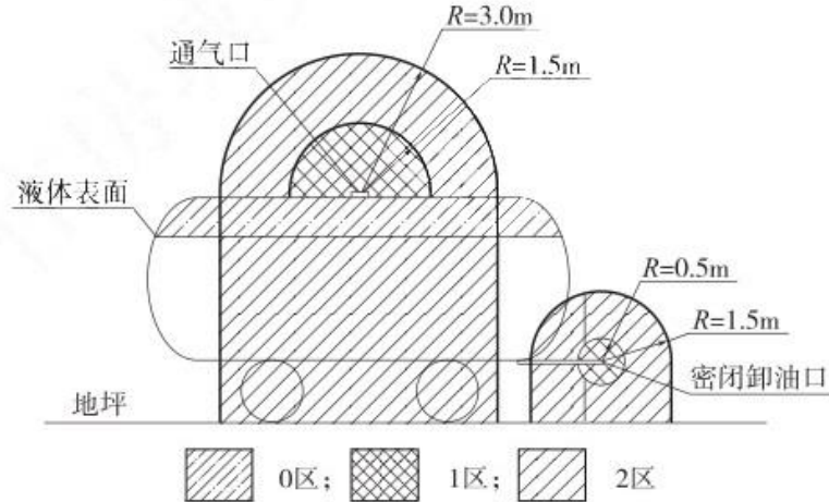
图 3-2 汽油油罐车的爆炸危险区域划分图
