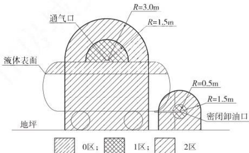
图 3-2 汽油油罐车的爆炸危险区域划分图
